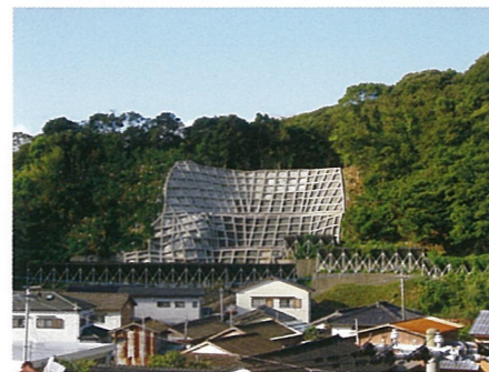
崩壊・落石対策工
